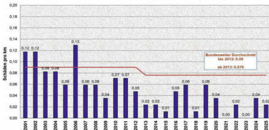
Diagramm 3 Schadensrate an Versorgungsleitungen im Versorgungsgebiet
